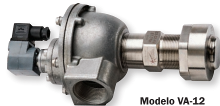
Modelo VA-12 (con válvula solenoide, acoplamiento de montaje y tuerca de fijación)
